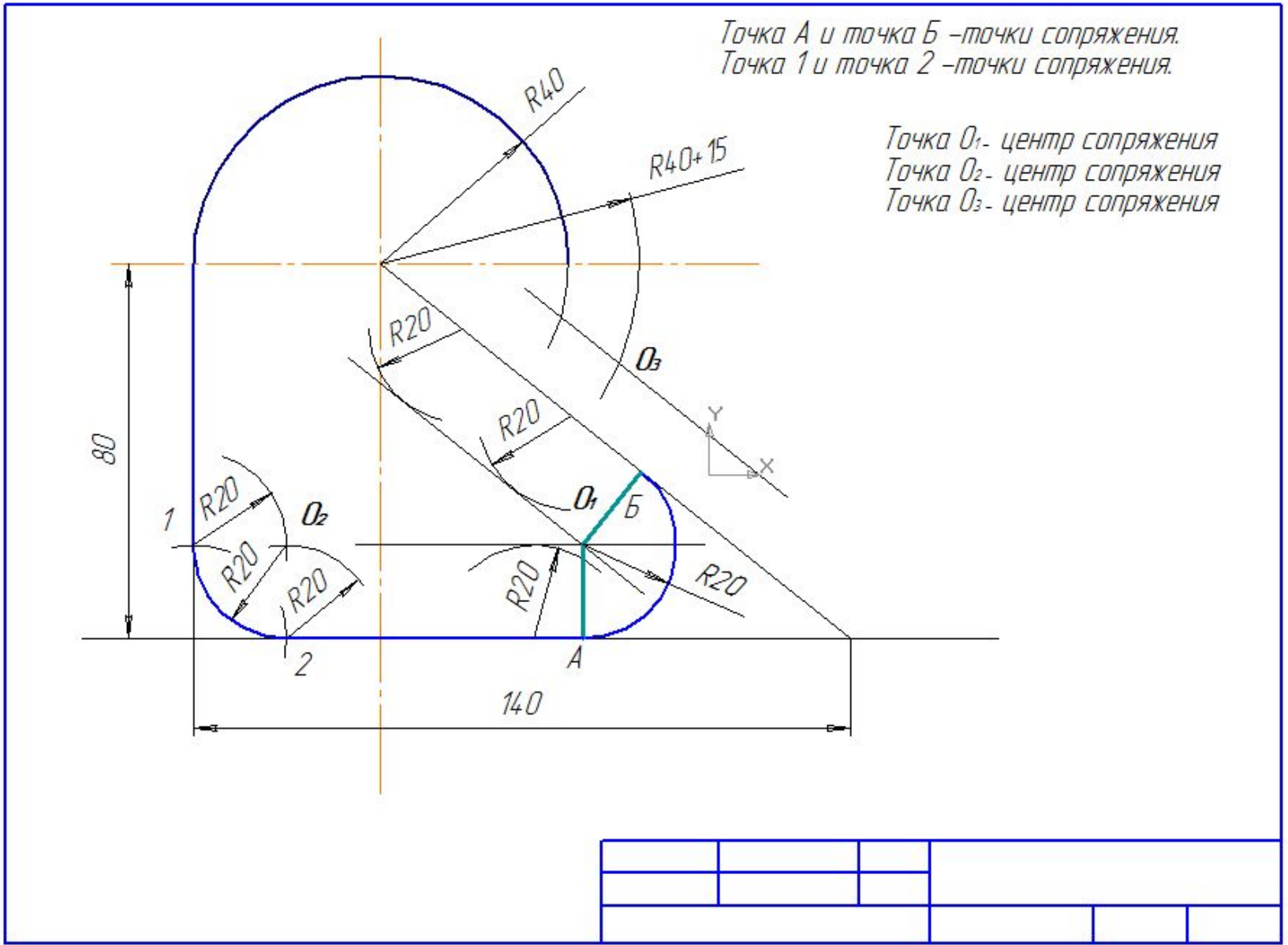
21. Стираем вспомогательные построения: дуги радиуса 15 мм.
