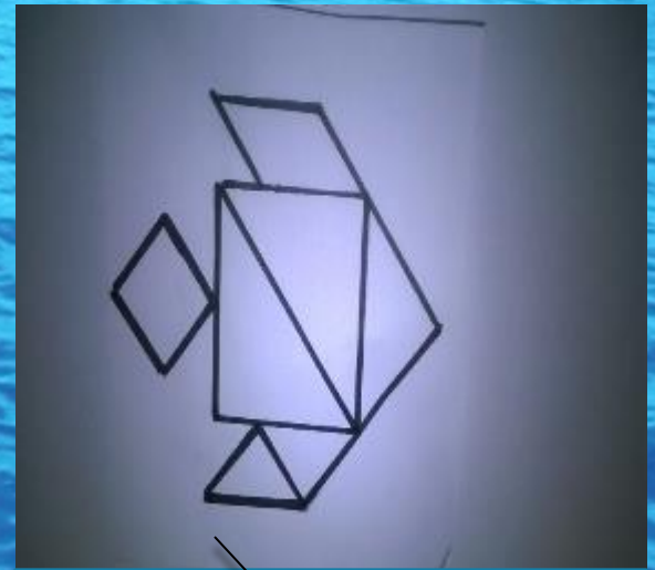
КАМБАЛА
