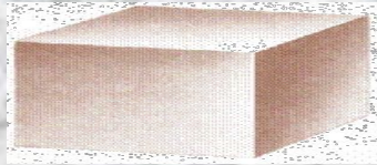
Гексаэдр
