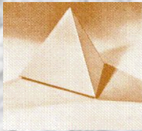
Тетраэдр
