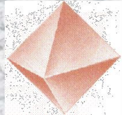
Октаэдр
