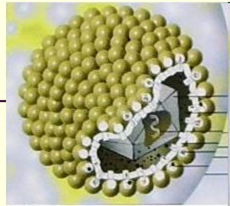
Строение цитомегаловируса
