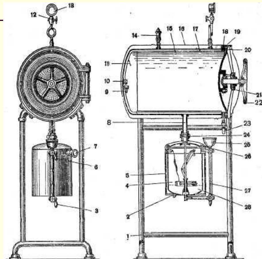
Рис. 1. Схема автоклава.
