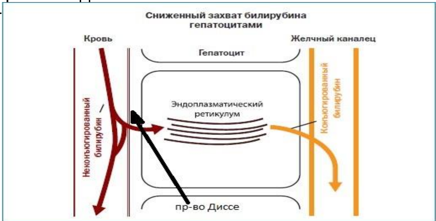
Рисунок 7. Патогенез синдрома Жильбера
