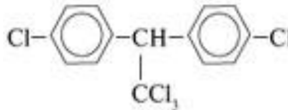
1,1,1-Трихлор-2,2-бис (p-хлорфенил)этан
