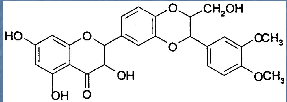
Силибин
