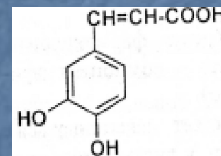
Кофейная кислота
