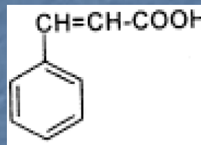
Коричная кислота
