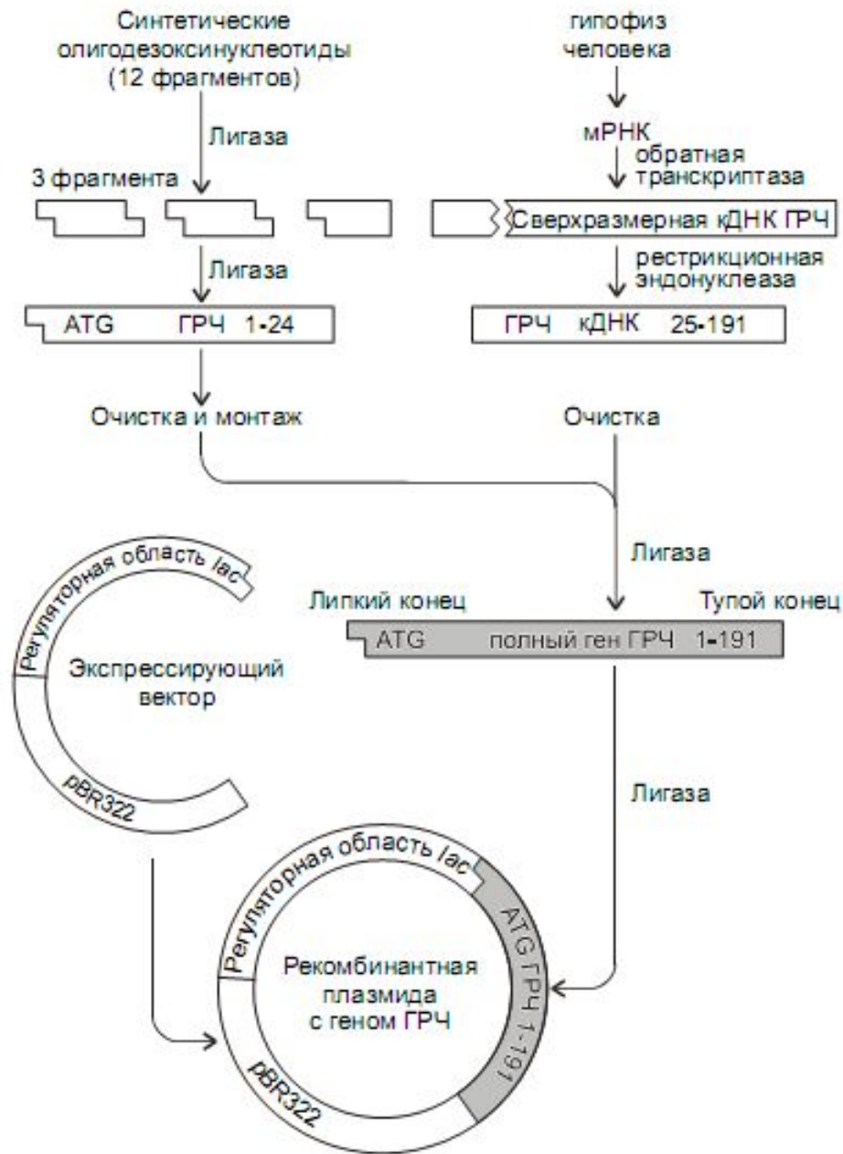
Рис. 4.4. Схема юнструирования гена соматотропина комбинацией химического синтеза и выделения природной мРНК (по Р. Newmark, 1979).
