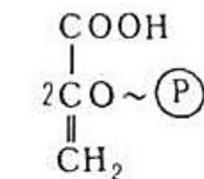
Фосфоенол-пировиноградная к-та
