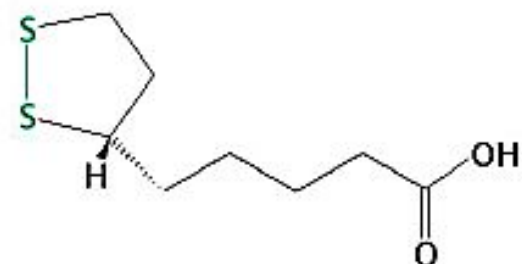
Липоевая кислота
