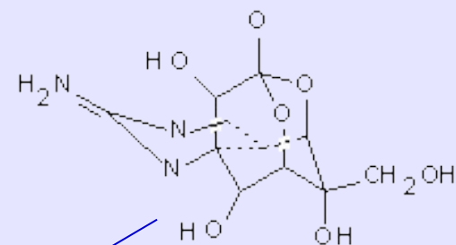
тетродотоксин рыбы
