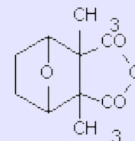
кантаридин жуки
