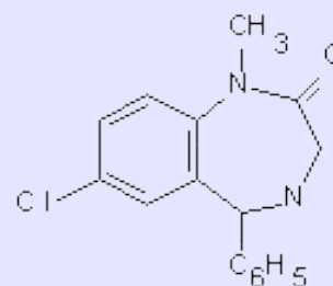
диазепам
