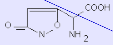
ибботеновая кислота
