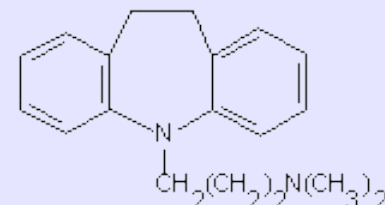
имипрамин
