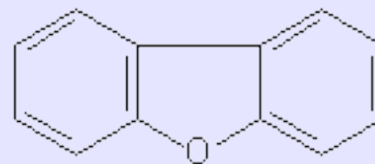
бензофуран
