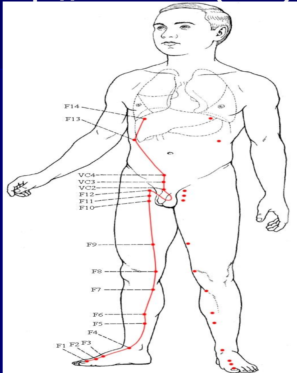
Рис. 18. Меридиан печени
