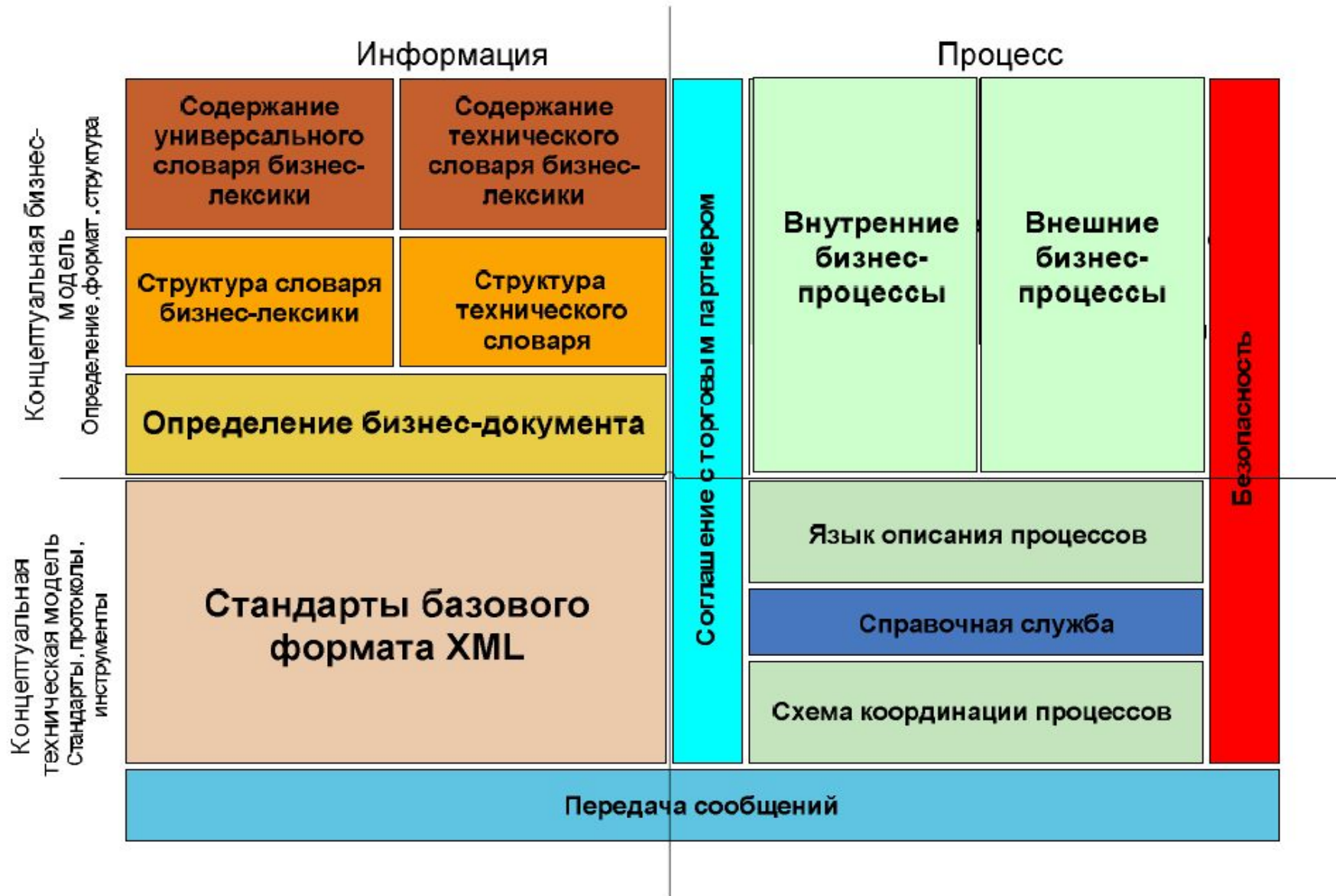
Концептуальная модель RosettaNet
