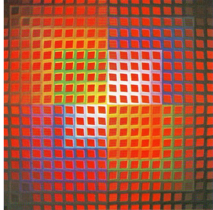
34. В. ВАЗАРЕЛИ. Сыновья II. 1966 г.
