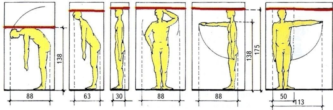
Параметры пространства при выполнении различных движений в положении стоя (для человека ростом 175 см)
