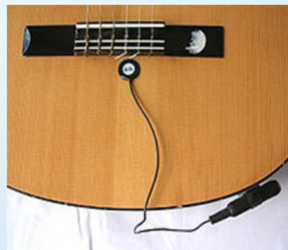
Пьезоэлектрический звукосниматель на классической гитаре
