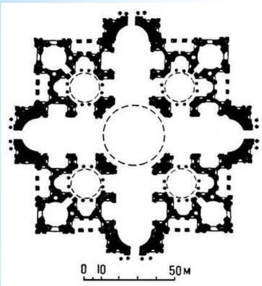
План собора св. Петра в Риме Архитектор Браманте
