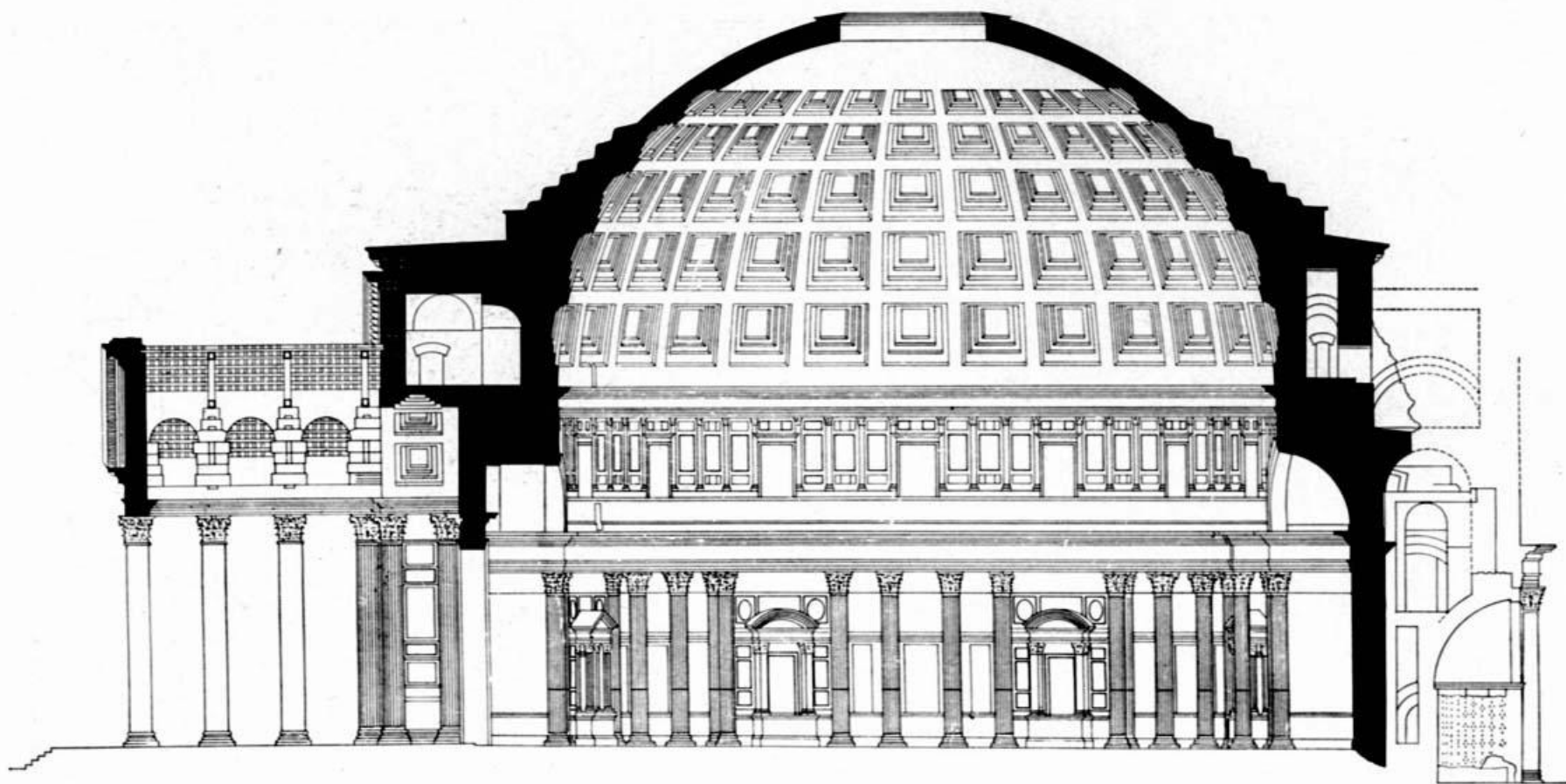
Пантеон. Около 125 г. Продольный разрез. Рим
