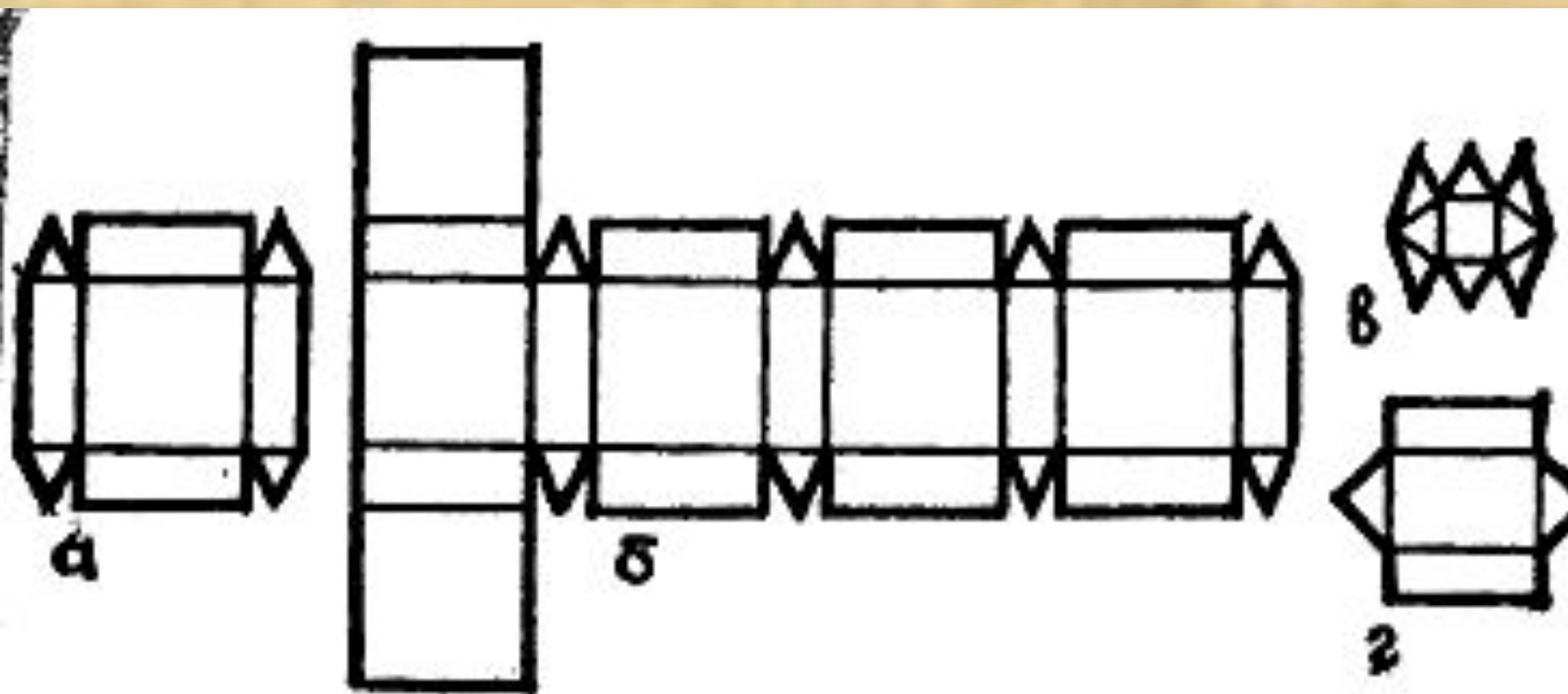
Рис. 7. Построение двадцатшестигранника — куба с усеченными ребрами: а — построение повторяющегося элемента развертки, б — полная развертка, в — построение развертки трехгранной призмы, г — развертка тела, сочленяемого с двумя первыми.
