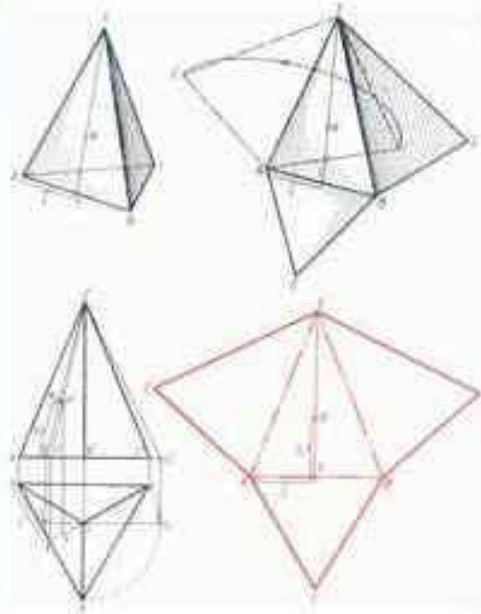
Развертка прямой трехгранной пирамиды
