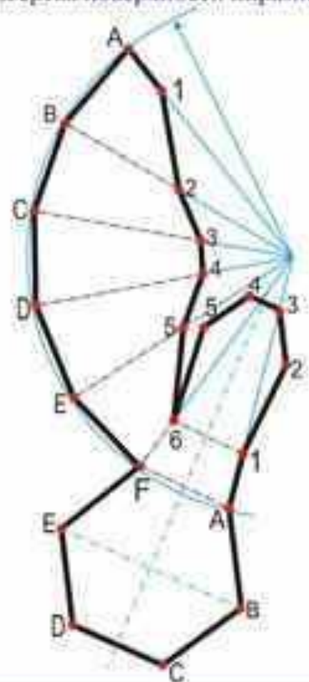
Развертка поверхности пирамиды
