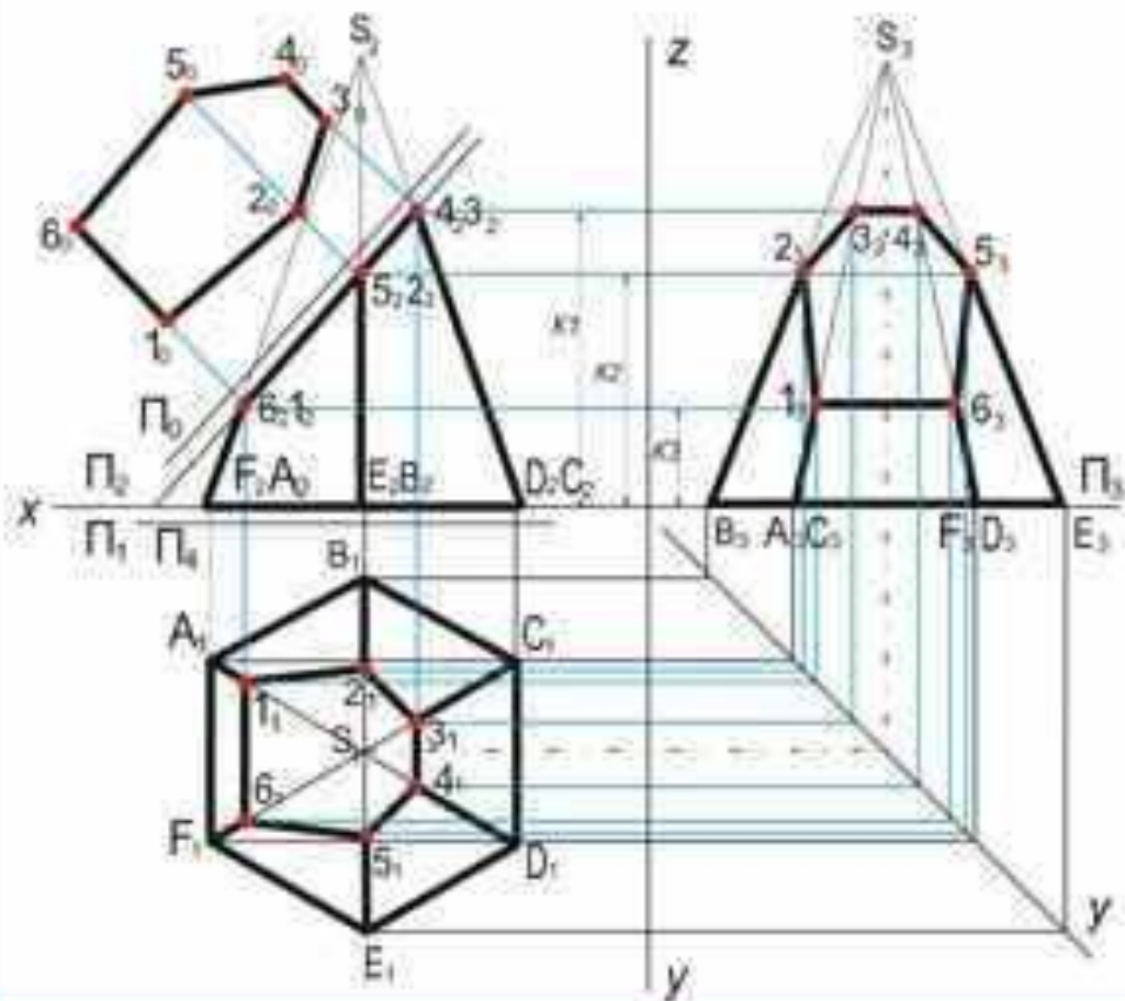
Сечение правильной шестиугольной пирамиды
