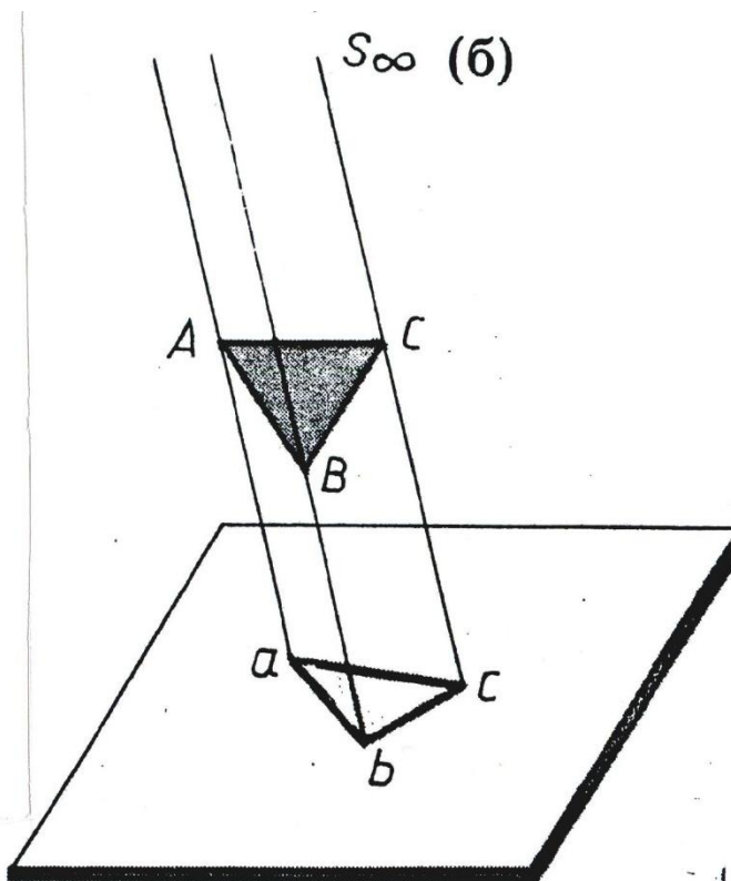
Параллельное проецирование
