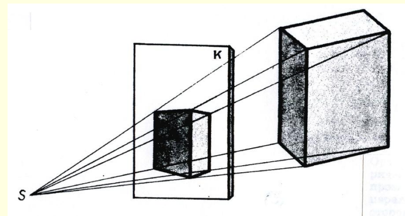
Центральное проецирование
