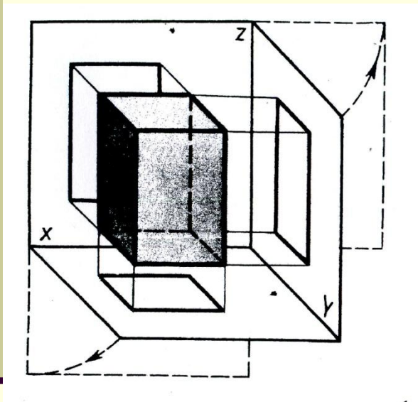
Ортогональное проецирование
