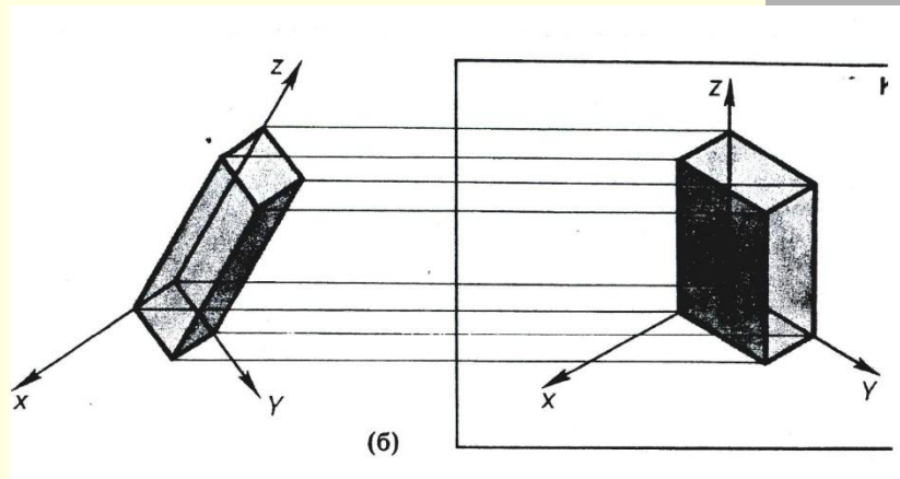
Параллельное проецирование (аксонометрическая проекция)
