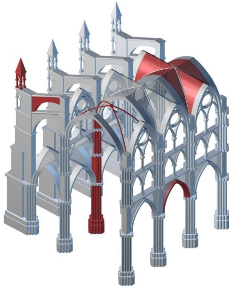
Готический храм. Схема
