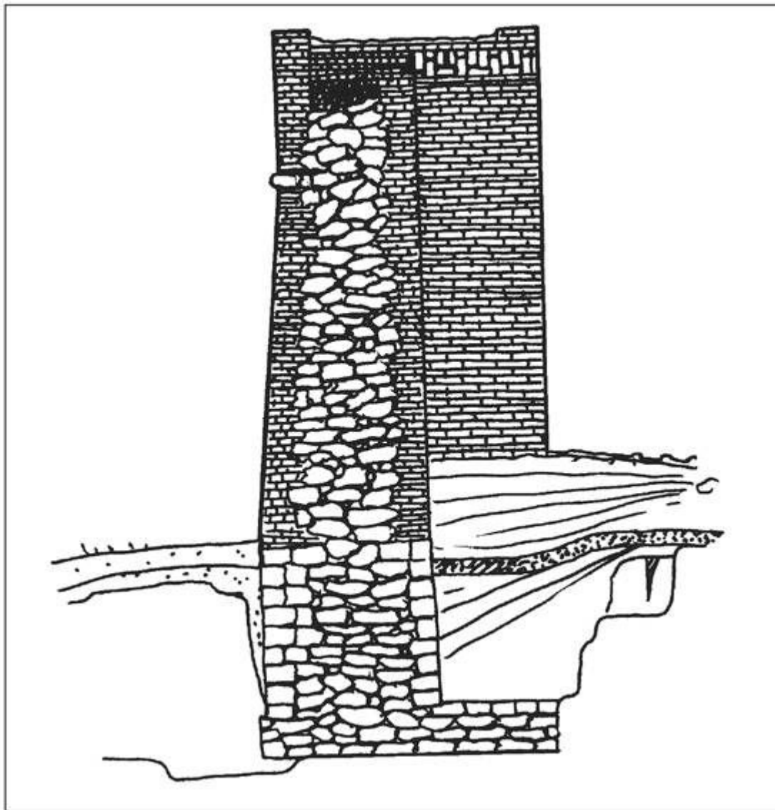
Полубутовая кладка. Северо-западная стена Нижегородского кремля
