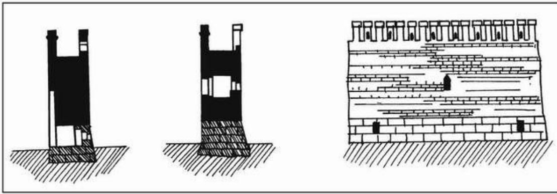
Устройство стен Смоленска, 1596 г.
