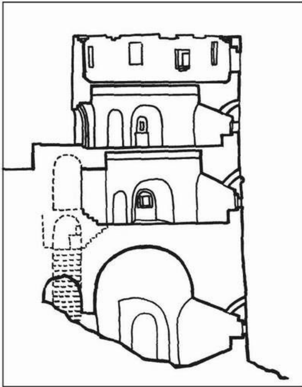
Тайничная башня Нижегородского кремля. Обратите внимание на дымоотводы
