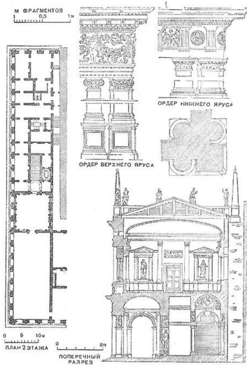
Венеция. Библиотека Сан Марко. Вверху — ее чертежи и торцовый фасад, внизу — библиотека и Лоджетта. Я. Сансовино
