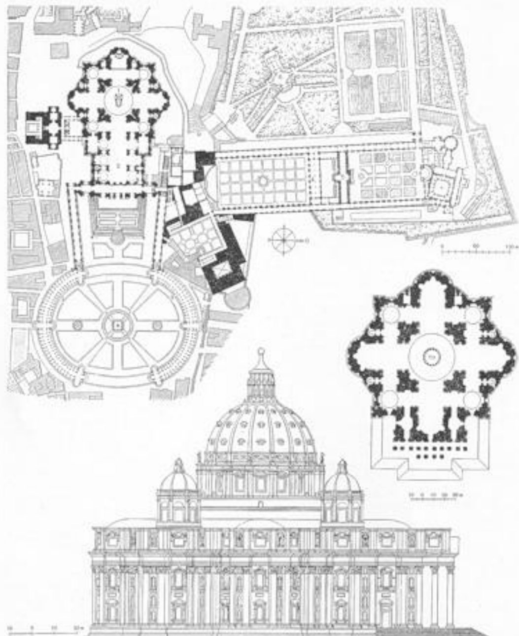
Рим. Ватикан и собор св. Петра, современное состояние. Внизу — план и фасад собора по проекту Микеланджело
