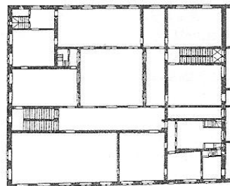
ПЛАН 2 ЭТАЖА
