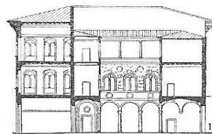
РАЗРЕЗ ПО ГЛАВНОМУ ВХОДУ
