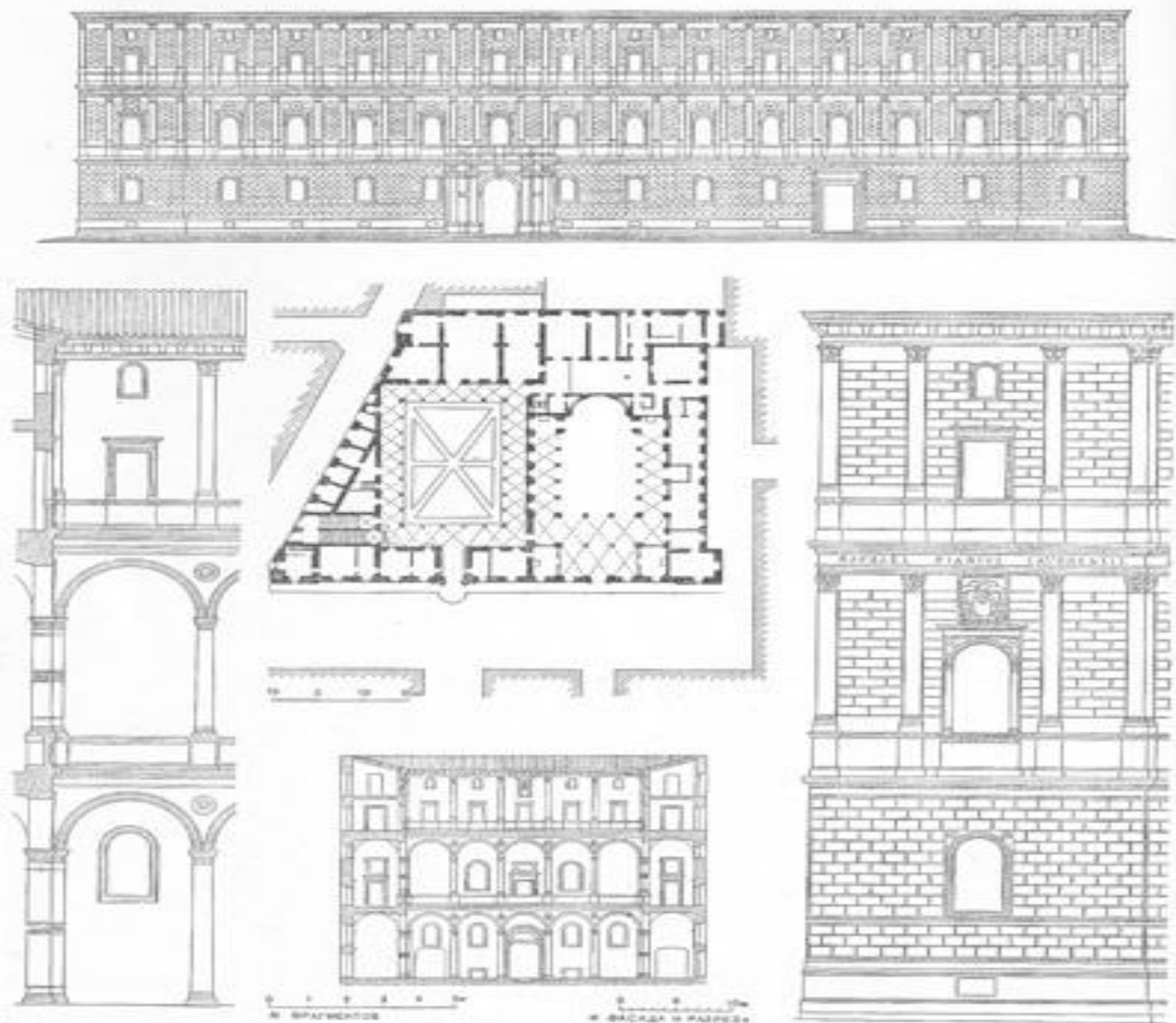
Рим. Палаццо Канцеллерия, 1483—1526 гг. Бренно, Браманте и др. (режисан по Летарун, до пробыаки Корсо Викторио-Эммануэле)
