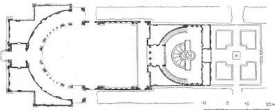
Рим. Вилла папы Юлия III, с 1550 г. Виньола, Вазари, Амманати и др.
