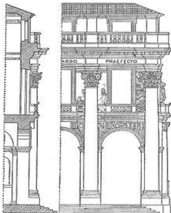
Палаццо дель Капитанио (Капитано) Виченца (Италия) с 1576г. Андреа Палладио Фрагменты разреза, главного фасада, его вид по проекту и торцовый фасад
