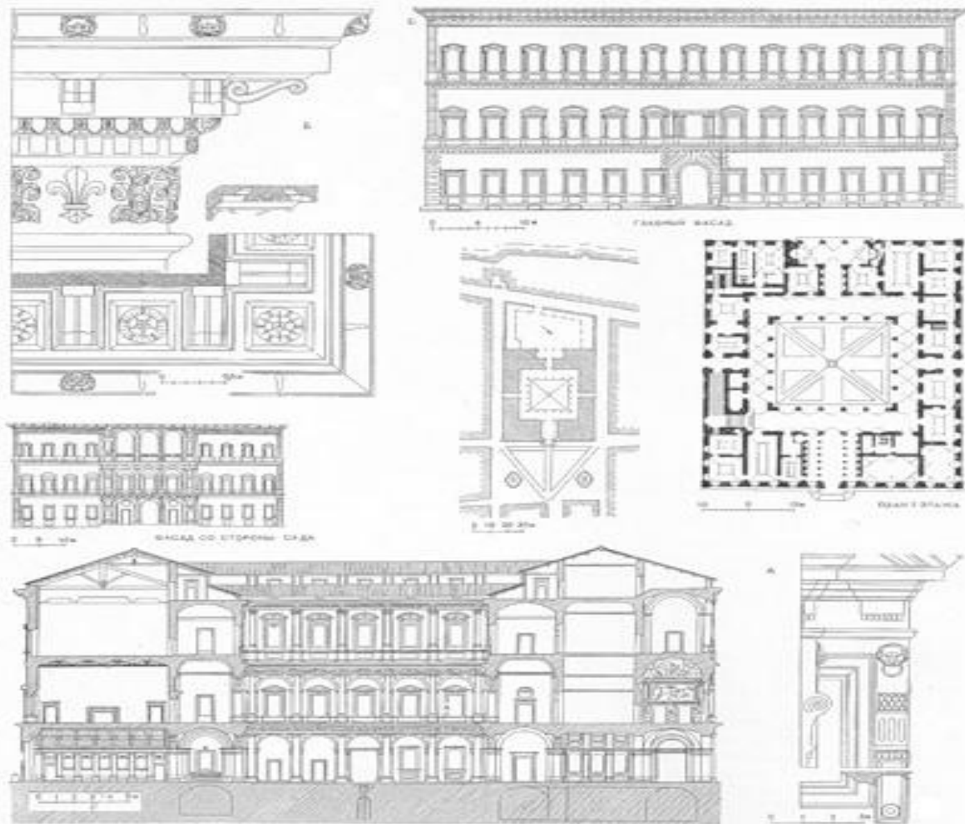
Рим. Палаццо Фарнезе, 1514—1589 гг. Антонио да Сангалло Младший, Микеланджело, Виньола, Джакомо della Porta
