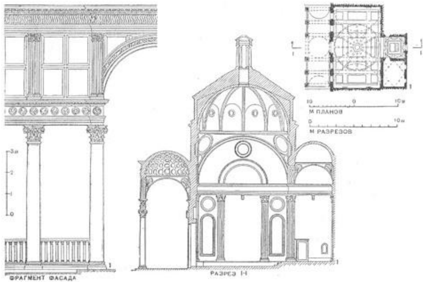
Капелла Пацци , Флоренция (Италия), 1456-1464гг., арх. Филиппо Брунеллеско
