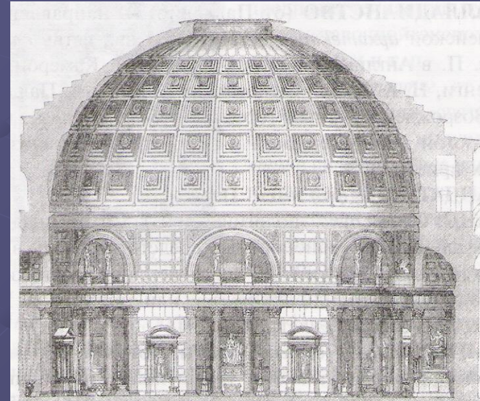
Разрез римского Пантеона. Реконструкция Адлера
