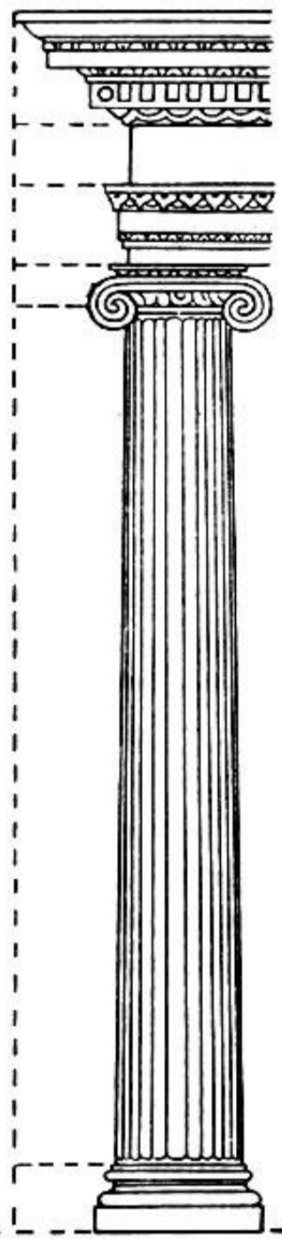
Ионический ордер
