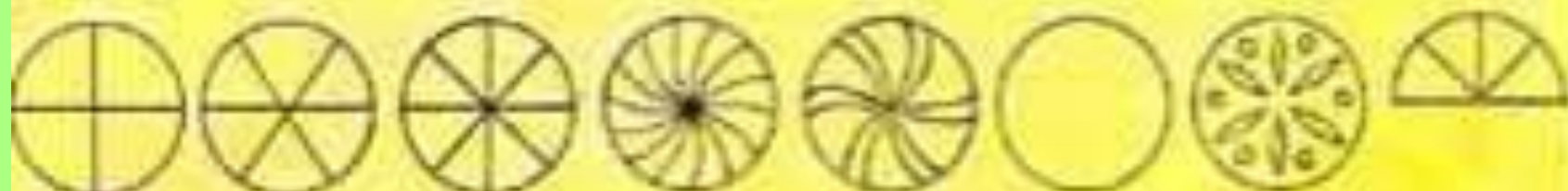
Солнце
