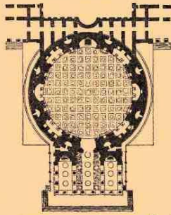
6. Планъ Пантеона Агриппы въ Римѣ.
