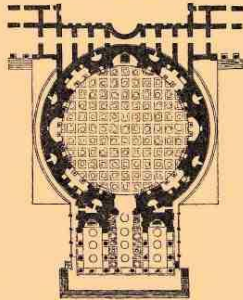
6. План Пантеона Агриппы в Риме.
