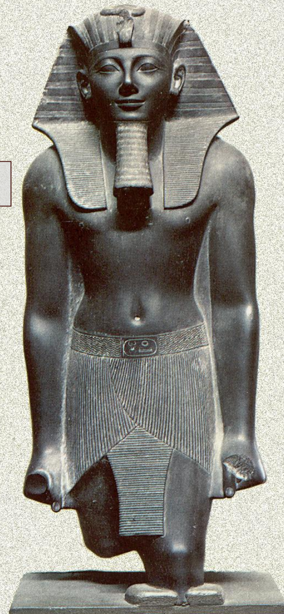
Базальт
