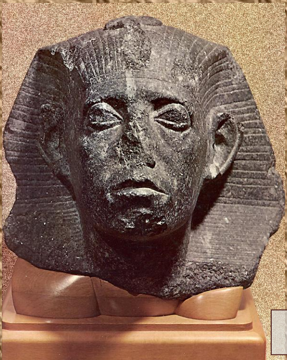
Гранит
