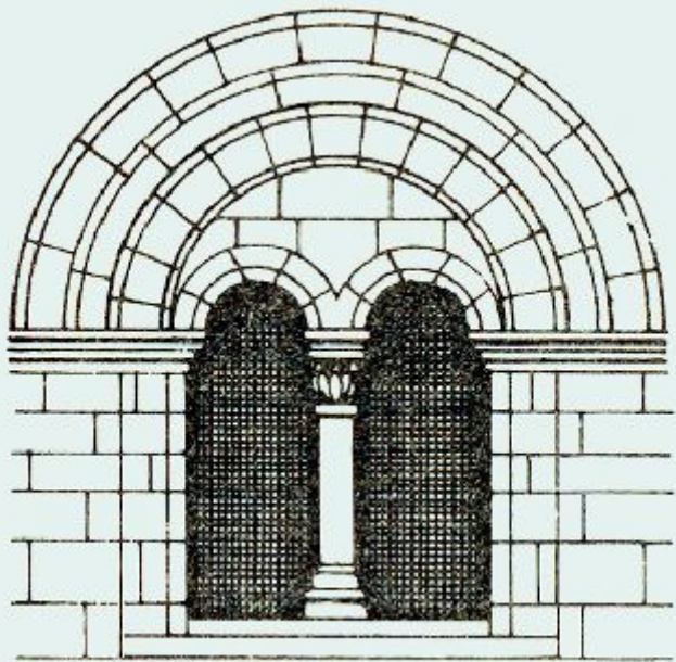
Романское двойное полуциркульное окно. Общая разгрузочная арка объединяет оконные проемы.
