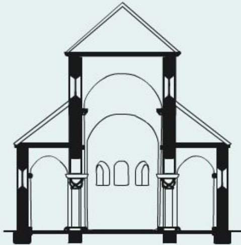
Романская базилика. Рисунок в разрезе.
