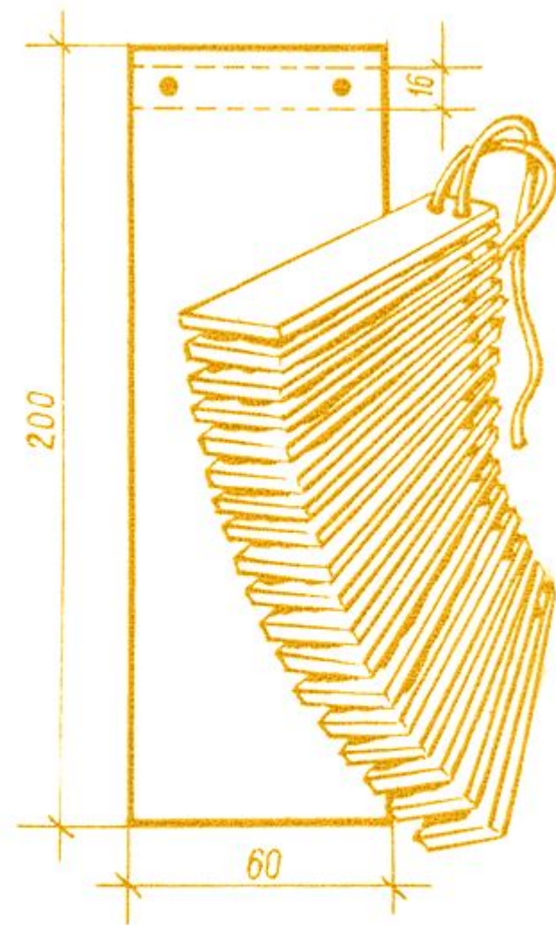
Общий вид трещотки и размеры ее пластин
