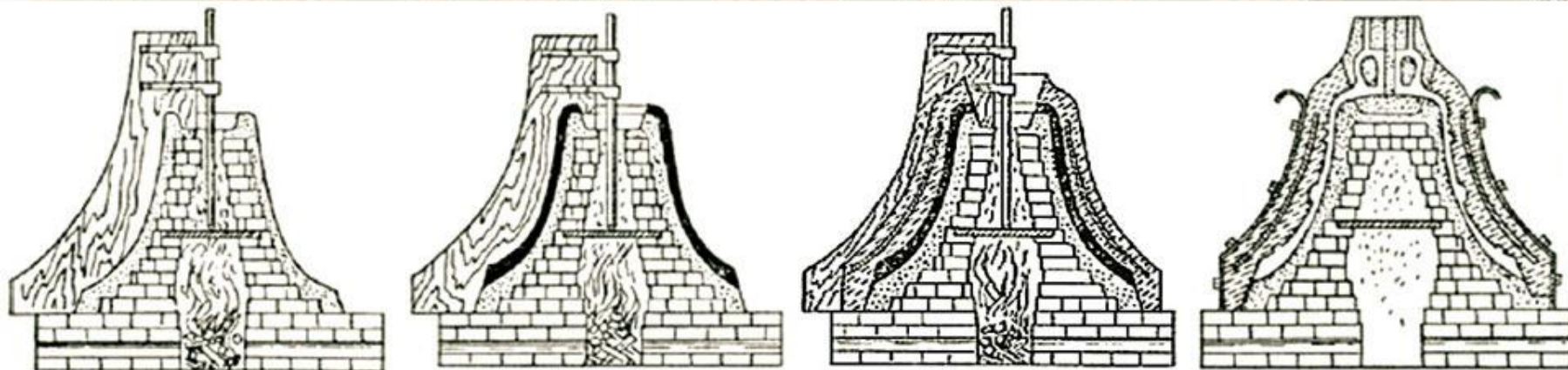
Стадии изготовления формы колокола согласно традиционной русской технологии.
