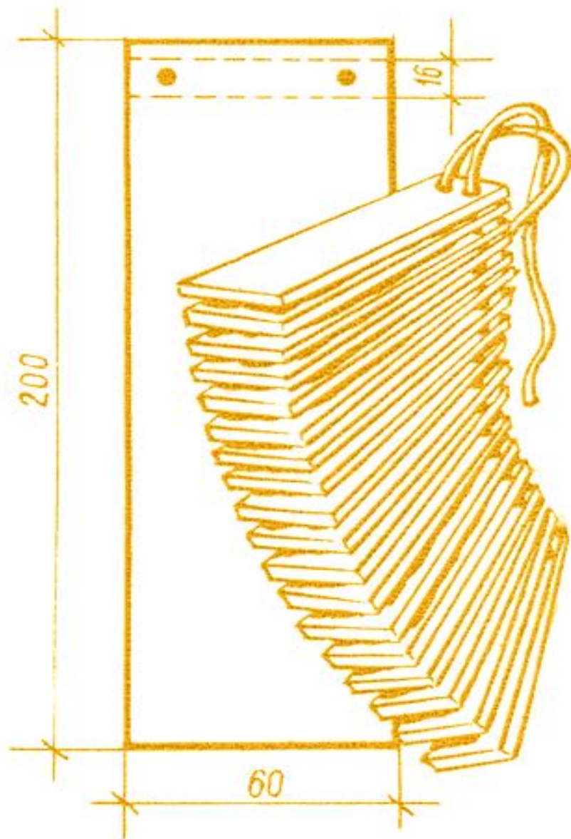
Общий вид трещотки и размеры ее пластин
