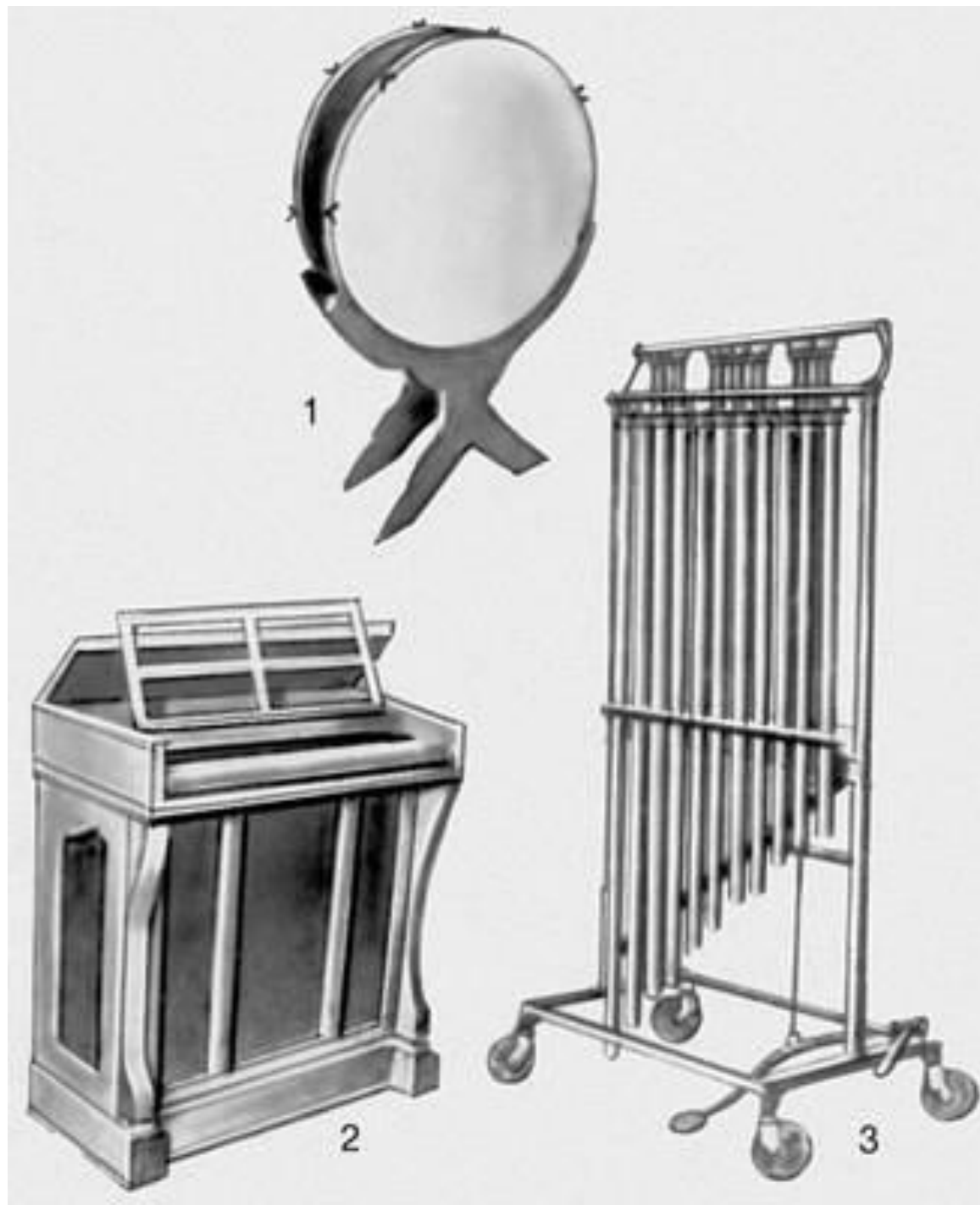
челеста
