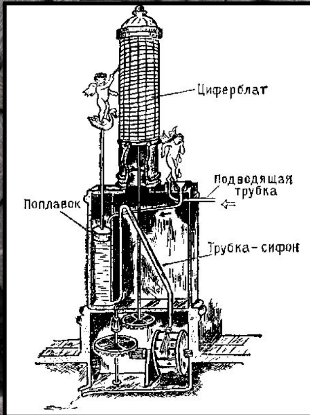
Водяные часы Ктезибия
