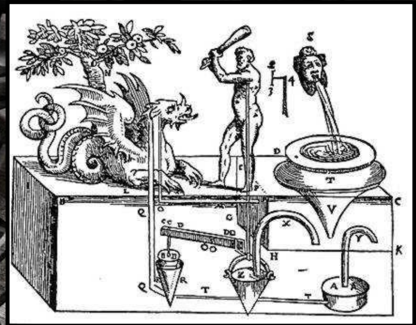
Механический театр Герона
