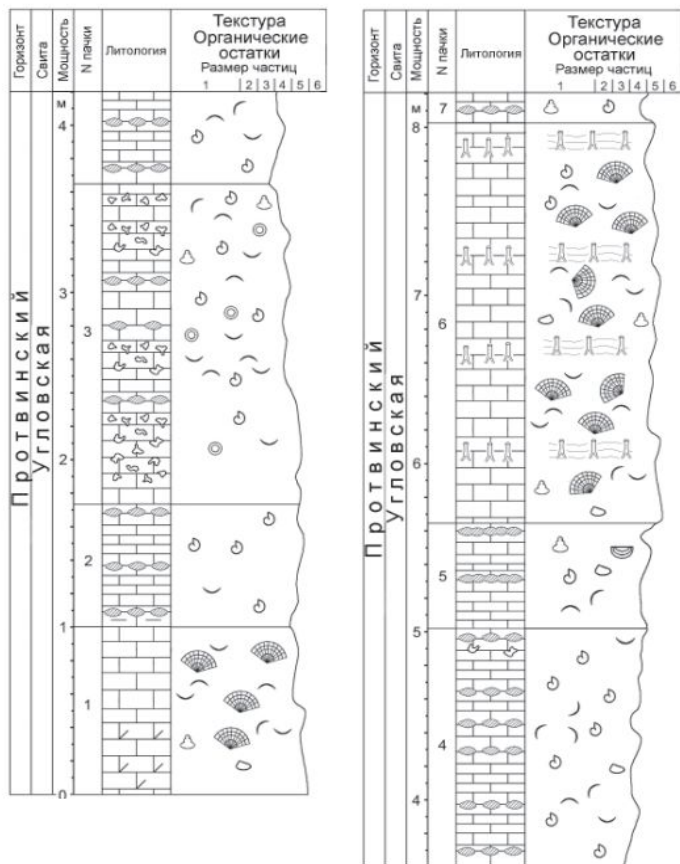
Опорный разрез нижнего карбона реки Мсты
