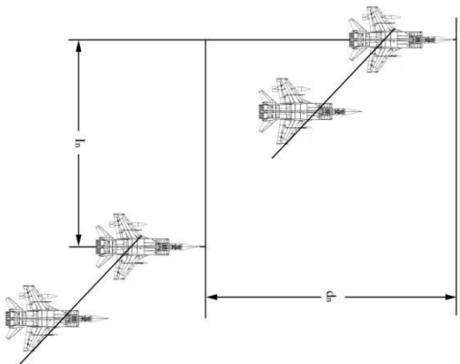
«пеленг пар»
