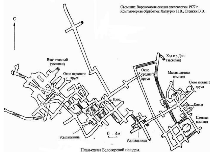
План-схема Белогорской пещеры.
