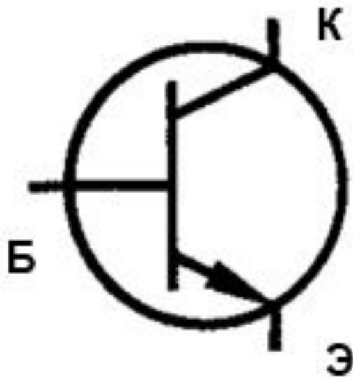
Биполярный NPN-транзистор
