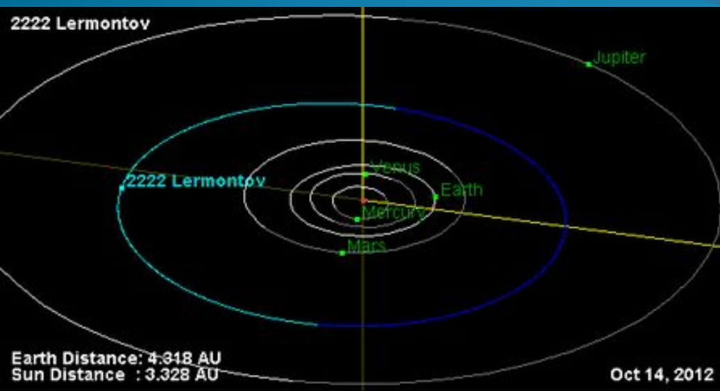
Орбита астероида Лермонтов и его положение в Солнечной системе
