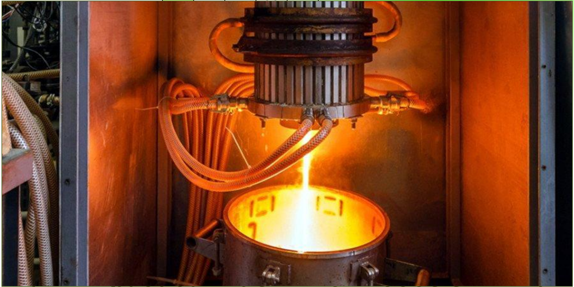
специальной вращающейся печке – кальцинаторе
