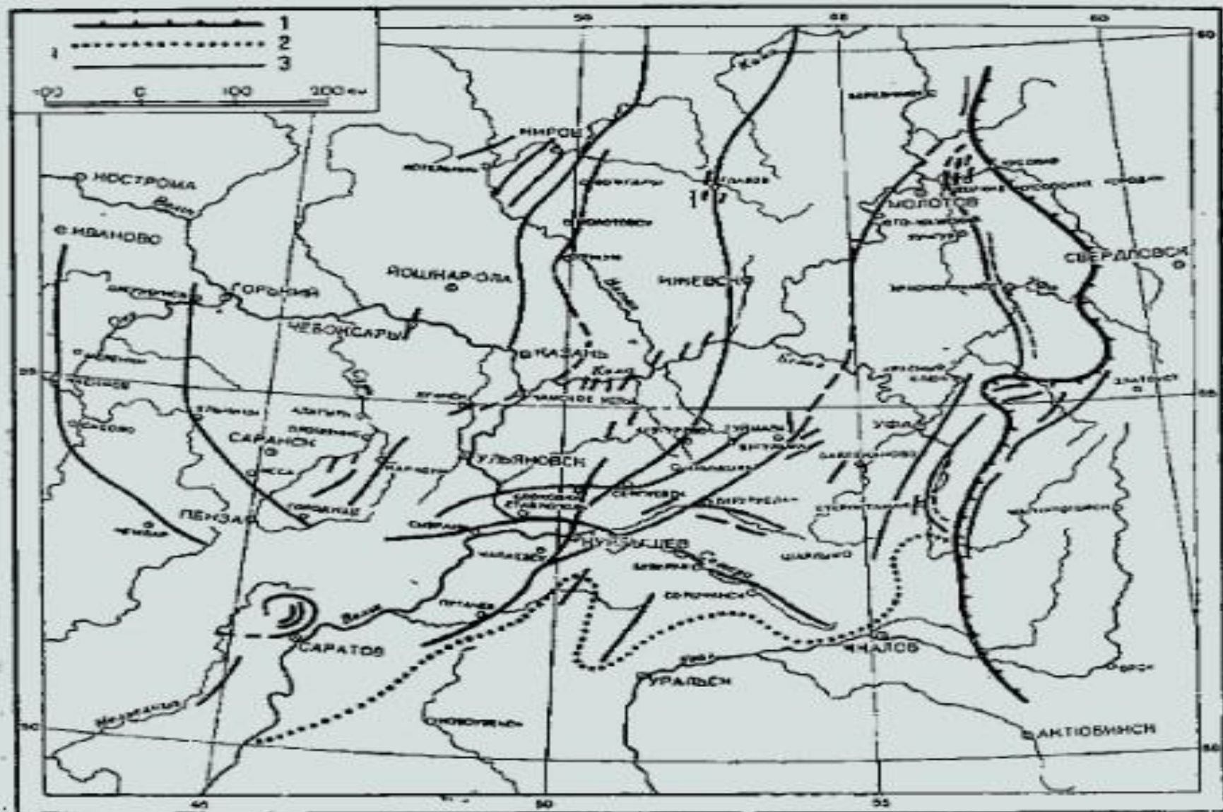
1-граница Уральской складчатой зоны; 2-граница области соляной тектоники; 3-тектонические линии.
