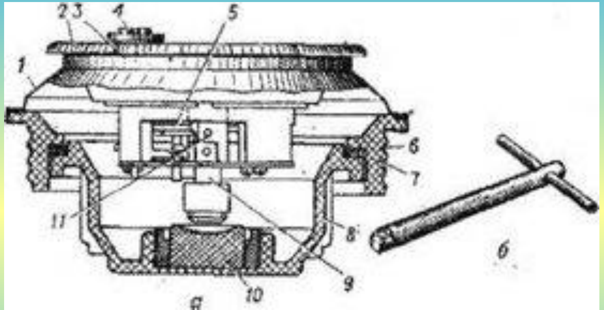
Разрез в боевом положении
