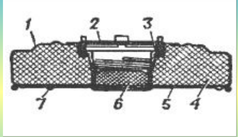
Разрез мины с пробкой
