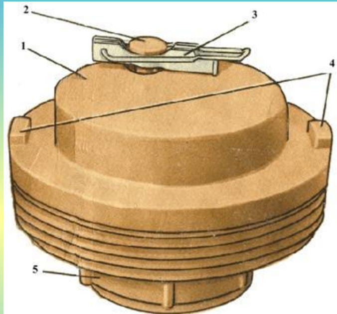
Взрыватель МВЧ-62
