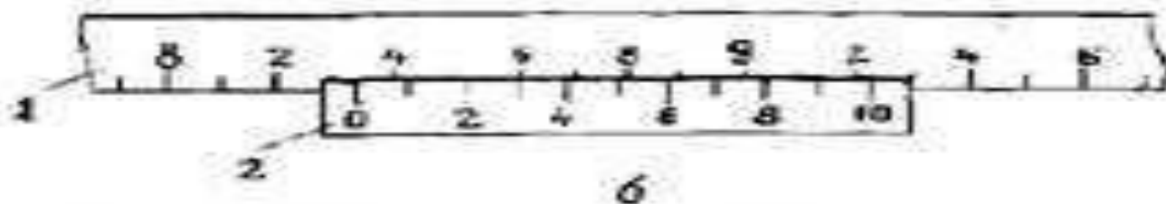
Рис. 16. Угломерное устройство Башенки: а — общий вид; б — шкалы; 1 — основная шкала; 2 — отсчетная шкала; 3 — указатель
