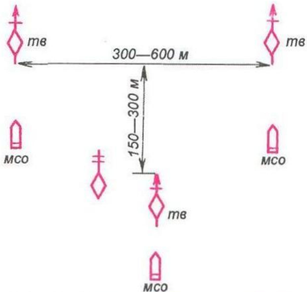
Рис. 6. Предбоевой порядок усиленной танковой роты. Положение танковых взводов — углом назад (вариант)
