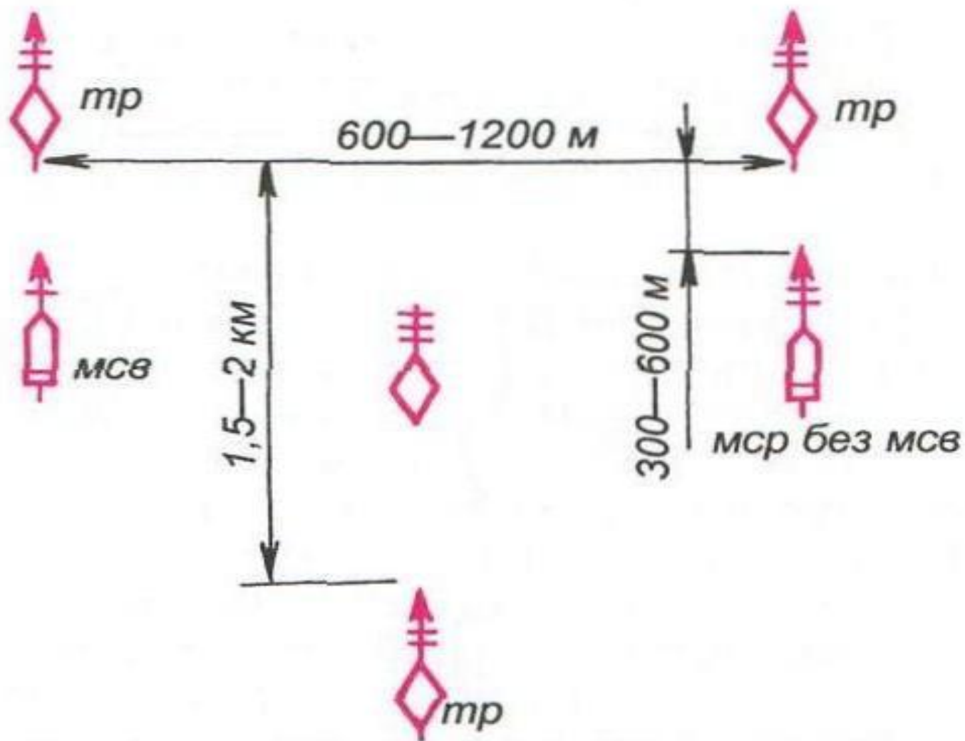
Рис. 4. Предбоевой порядок усиленного танкового батальона ротными колоннами. Положение танковых рот — углом назад (вариант)
