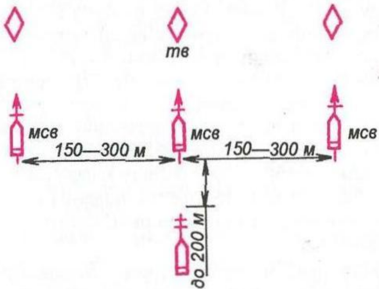
Рис. 5. Предбоевой порядок мотоциклетной роты. Положение мотоциклетных взводов — в линию колонн (вариант)
