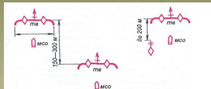
Рис. 10. Боевой порядок усиленной танковой роты. Положение взводов — углом назад (вариант)
