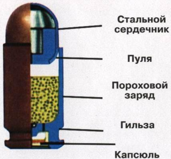
Общий вид 9-мм пистолетного патрона и его устройство
