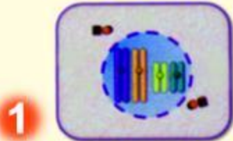
МЕТАФАЗА 1
