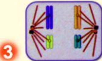
ТЕЛОФАЗА 1
