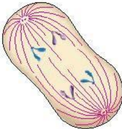
Анафаза
