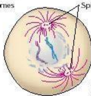
Профаза
