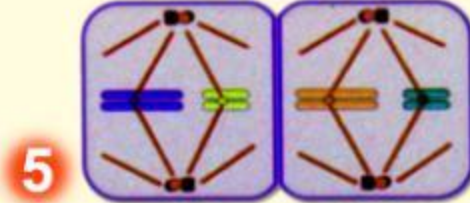
МЕТАФАЗА 2
