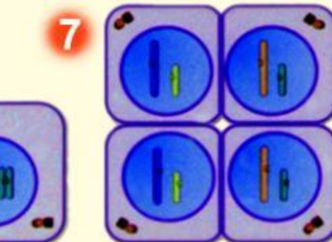
ТЕЛОФАЗА 2
