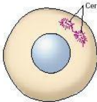
Интерфаза ( G_2 )
