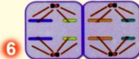
АНАФАЗА 2
