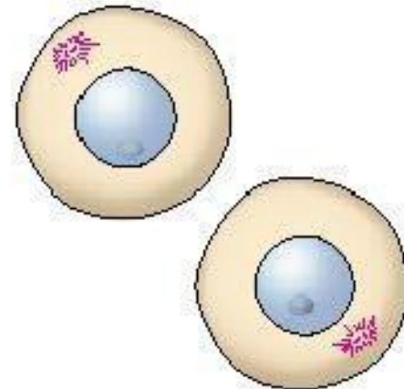
Интерфаза ( G_2 )
