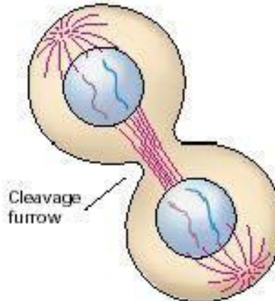
Телофаза
