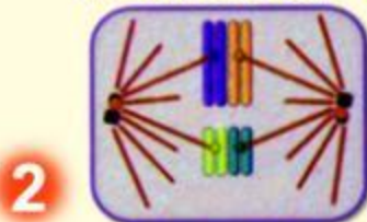
АНАФАЗА 1
