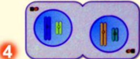
ТЕЛОФАЗА 1
