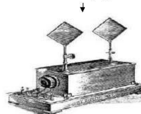
● Когерер
