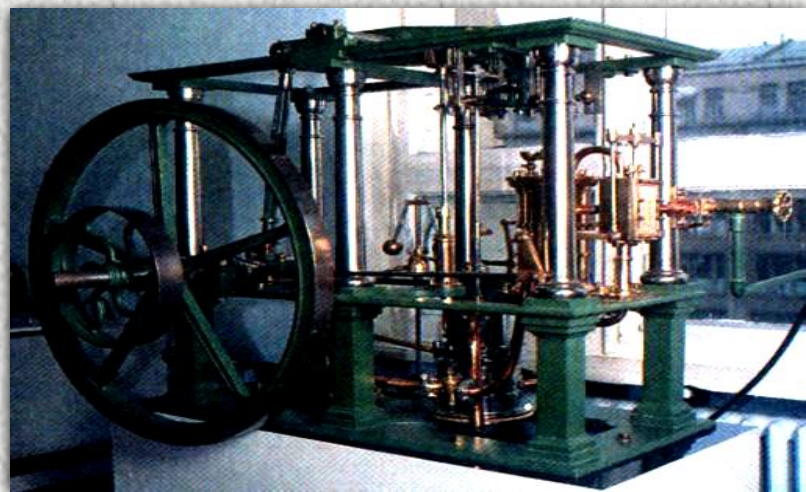
Паровая машина Дж. Уатта.
