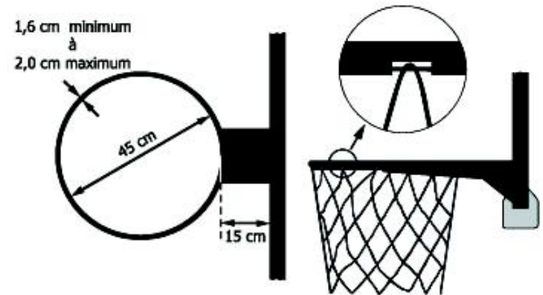
Figure 8 Anneau réglementaire
