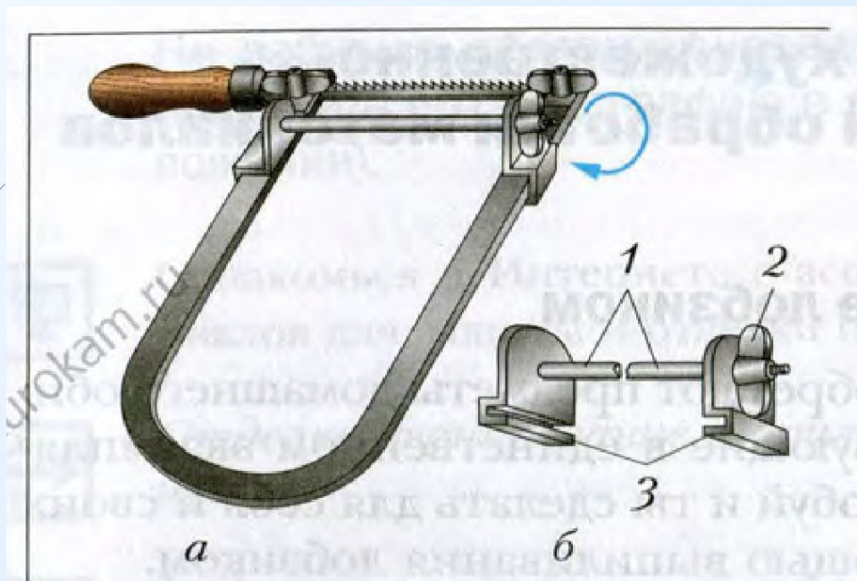
Рис. 69. Закрепление пилки в лобзике (а) и приспособление для стяжки концов рамки (б): 1 — резьбовая шпилька; 2 — гайка; 3 — стяжка
